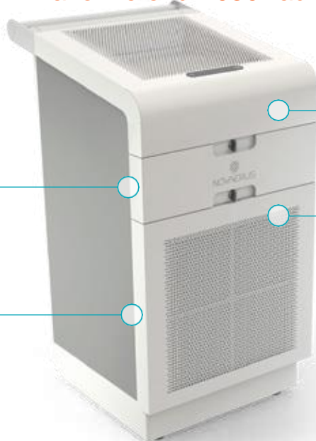
G4 UGLJIČNI FILTER Aktivirani ugljični filter Camfil® absorbira VOC, mirise i nečistoće
